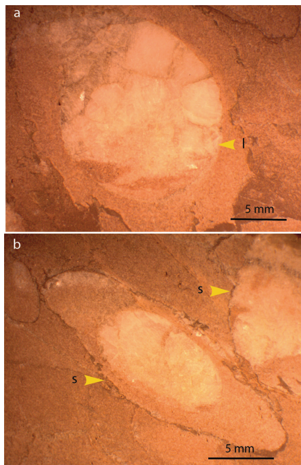
Fig. 11 a et b. Belloc (Villefranche-de-Conflent, Pyrénées-Orientales) carrière haute dans le marbre griotte. Déformations des restes de goniatites. En a : recristallisation en calcite sparitique blanche d'un test de goniatite (disque blanc en œil de perdrix), le contour général de la coquille est bien conservé ainsi que le dessin de quelques loges (l). En b : volume du test dont le disque blanc central a été étiré sous la pression tectonique, le pourtour externe étant souligné par un joint stylolithique (s). DAO. Pierre Giresse © Université de Perpignan-Via Domitia.
