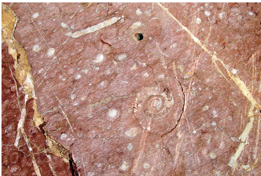
Fig. 1. Noves de Segre (Province de Lleida, Généralité de Catalogne), cantera del coll de Mu. Aspect macroscopique d'un rare fossile de goniatite assez bien conservé sur un bloc scié au câble dans le beau marbre griotte d'une carrière logée à 1 200 m d'altitude dans la Serra de Prada Castellà, en Urgellet, et qui a été récemment fermée ; longueur maximale du fossile 6 cm. Michel Martzluff © Université de Perpignan-Via Domitia.
