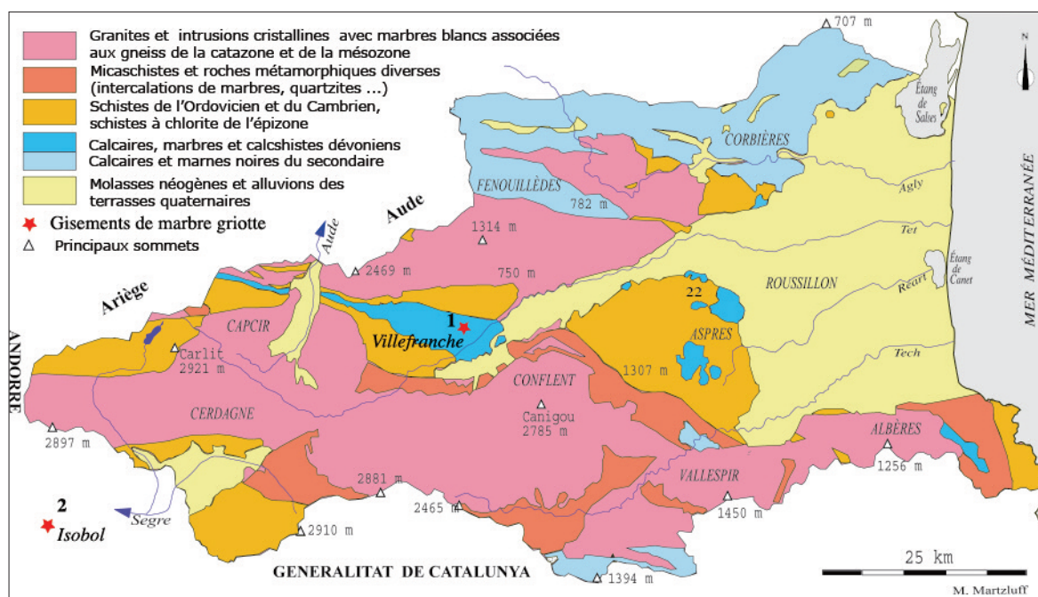
Fig. 3. Localisation des affleurements de marbre griotte du Conflent et de Cerdagne. N°1 : affleurements du Famennien inférieur (niveau D5b-6 de la carte géologique de Prades au 1/50 000, BRGM) dans le synclinal de Villefranche-de-Conflent, P.-O., carrières de Belloc et Roca fumada. N°2 : affleurements du Frasnien-Famennien (niveau DsB de la carte géologique de Saillagouse au 1/50 000, BRGM) en Cerdagne, carrière d'Isolbol. DAO. Michel Martzluff © Université de Perpignan-Via Domitia.
