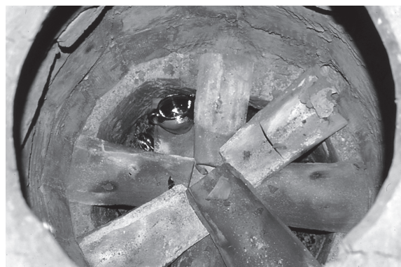
Fig. 9 : Four médiéval B, sole du four en tuiles canal après cuisson enfumée (cl. J.-M. Giorgio).
