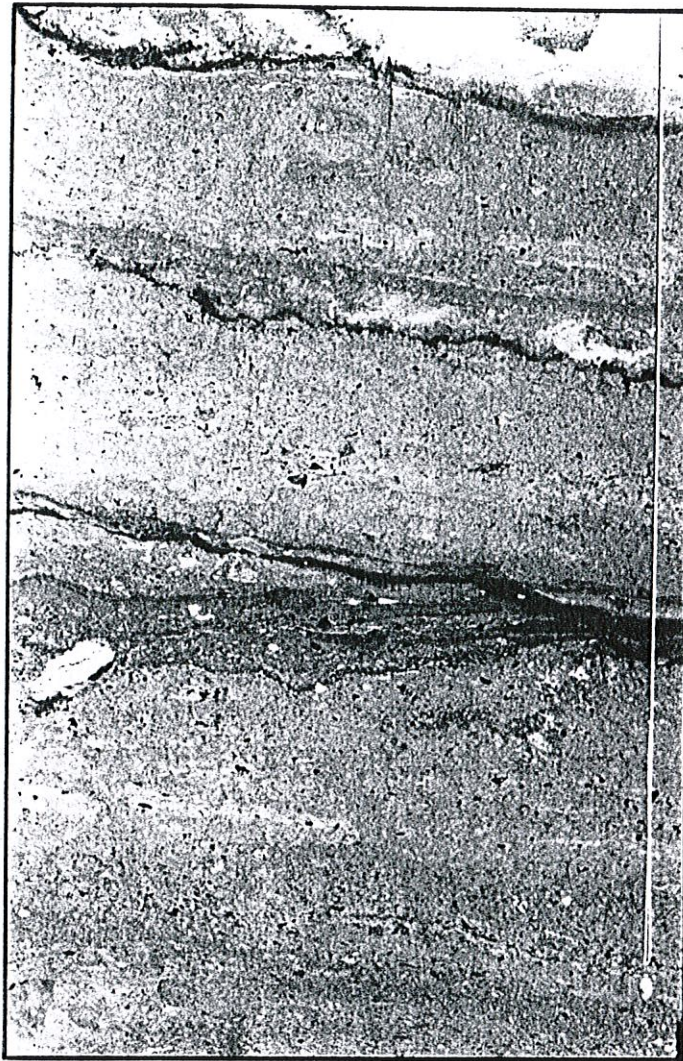
Bélesta - Salle la - Coupe stratigraphique (hauteur 1,50 m) des niveaux néolithiques final et moyen présentant des strates de brûlage (cl. F. Claustre)
