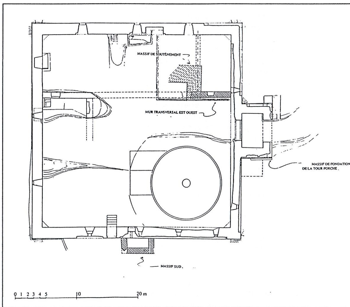
QUILLAN, Château - État des dégagements en 1995 (relevé M. Verrot)
